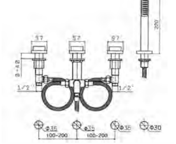
Movimenti ceramici/ Ceramic discs valves 19W
