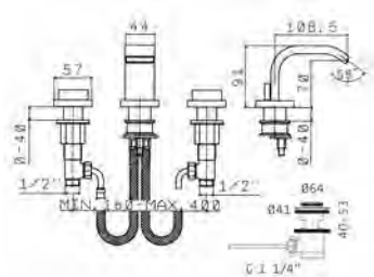
Movimenti ceramici/ Ceramic discs valves 19W
