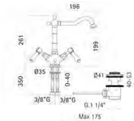
Movimenti ceramici/ Ceramic discs valves 29M
