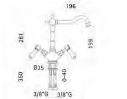
Movimenti ceramici/ Ceramic discs valves 29M
