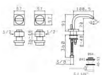
Movimenti ceramici/ Ceramic discs valves 19W
