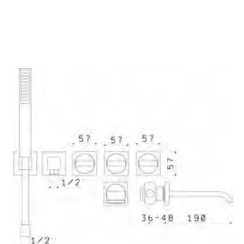
Movimenti ceramici/ Ceramic discs valves 19W
