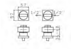
Movimenti ceramici/ Ceramic discs valves 19W
