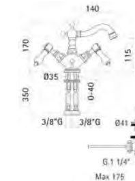
Movimenti ceramici/ Ceramic discs valves 29M
