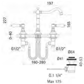
Movimenti ceramici/ Ceramic discs valves 29M
