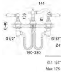
Movimenti ceramici/ Ceramic discs valves 29M
