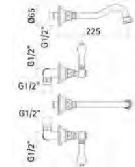
Movimenti ceramici/ Ceramic discs valves 29M
